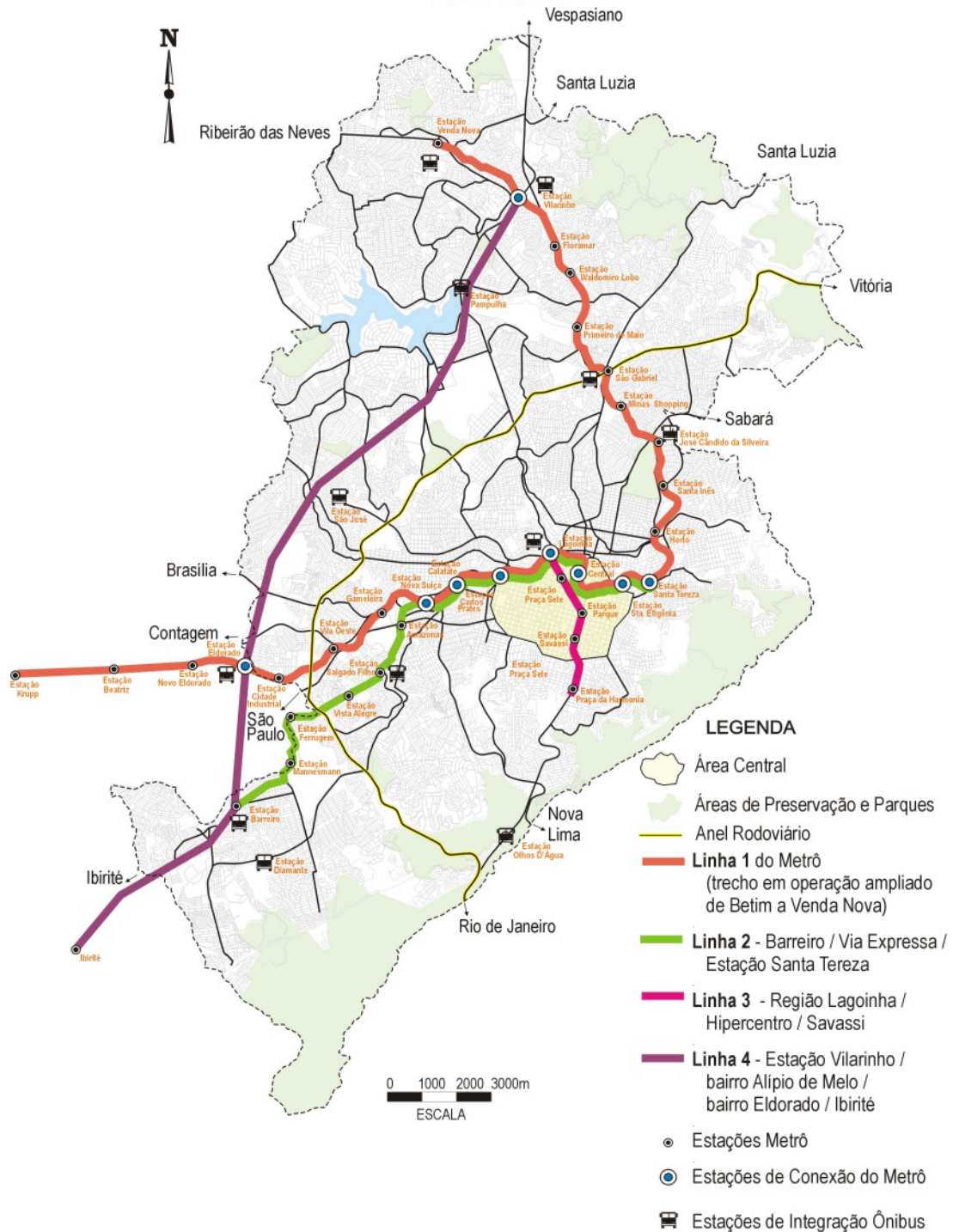
FIGURA 24 - Representação gráfica do Cenário escolhido para implantação do Plano Diretor de Transporte de Passageiros Sobre Trilhos da RMBH – Cenário 6 Fonte: INECO, 1999.
