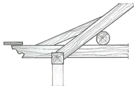
Figura 4: Beiral encachorrado
