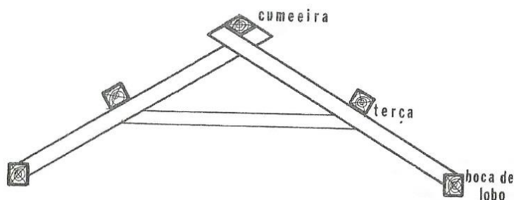
Figura 3: Cumeeira. (VASCONCELLOS, 1979)
