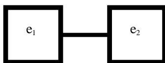
FIGURA 3 – Diagrama simbolizando a estrutura semântica de uma preposição
