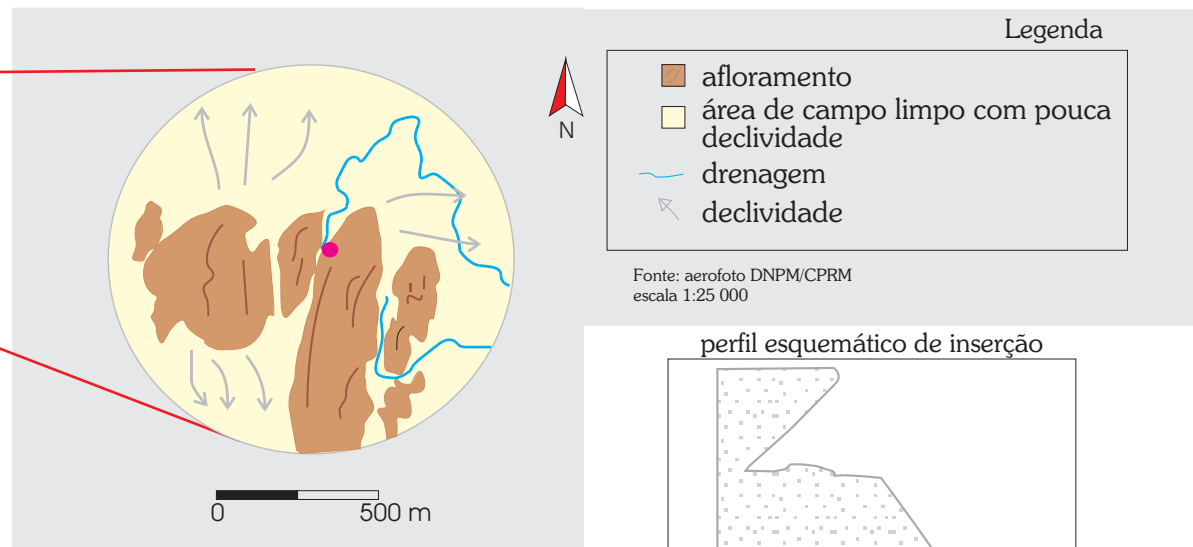
croquis esquemático de planta baixa do abrigo
