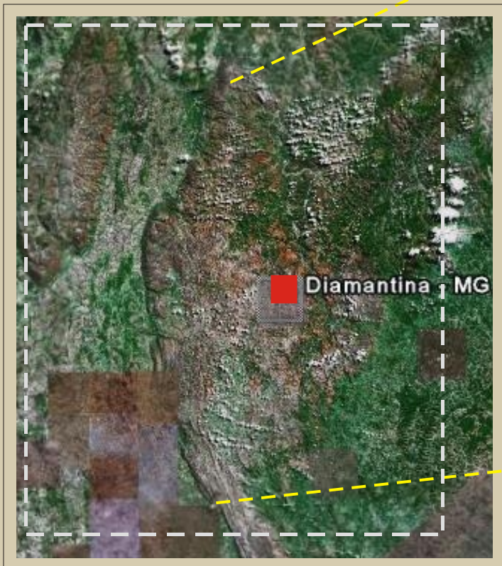
Mapa de localização da Região do Antigo Distrito Diamantino no Planalto meridional da Serra do Espinhaço
