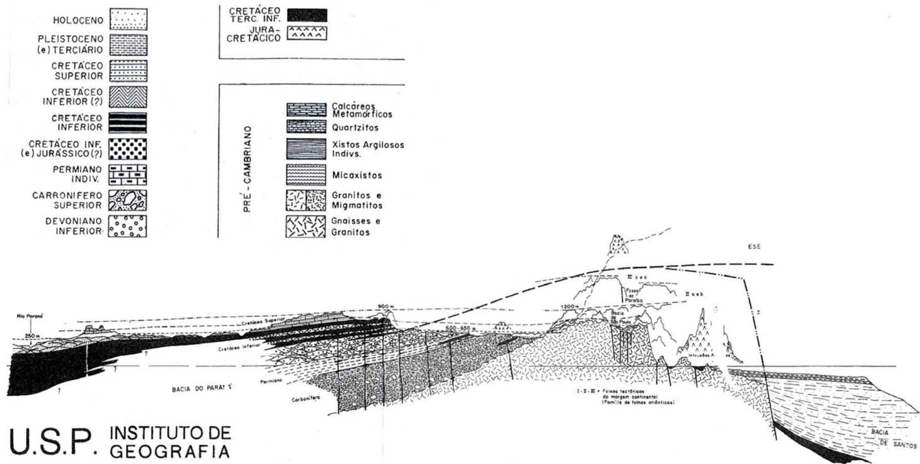
Figura 02 - Corte transversal do interior para a borda da bacia sedimentar do Paraná, sentido SW-NE, em que se verifica a posição da depressão periférica paulista dentro da qual se situa a cidade de Piracicaba e a área estudada. Escala 1 : 500 000. Fonte: IG / USP (1982).
