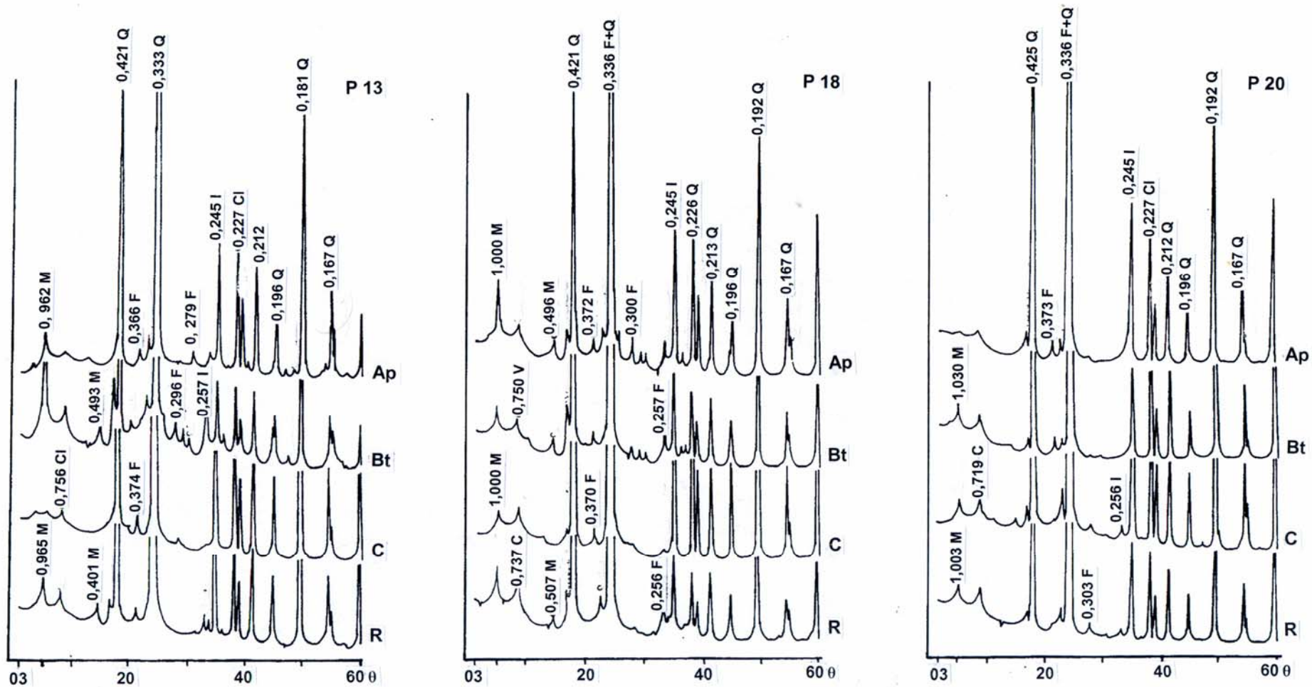
Figura 10 - Difratomogramas de raio x relativos á fração silte dos horizontes Ap, Bt e C, e ao saprólito Cr dos perfis 02 (P 13), 03 (P 18) e 04 (P 20) estudados. M = muscovita; Cl = clorita; Q = quartzo; F = feldspato; V = vermiculita e I = illita.
