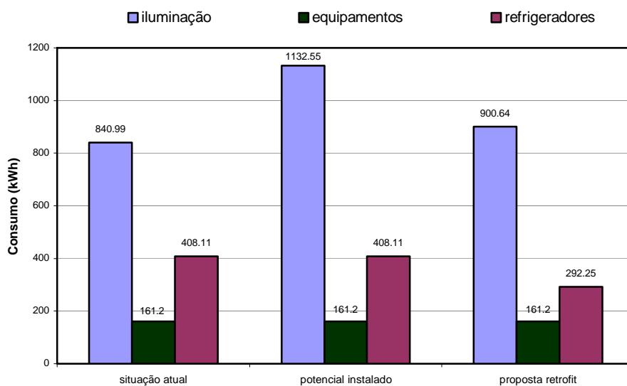
GRÁFICO 09: Comparativo do consumo desagregado para a sit. atual, pot. instalado e a prop. de retrofit .
