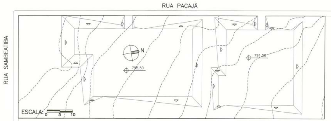
FIGURA 22: Planta de Movimento de Terra da Escola E. Pero Vaz. FONTE: Elaborado pela autora a partir de levantamento realizado em agosto de 2005.
