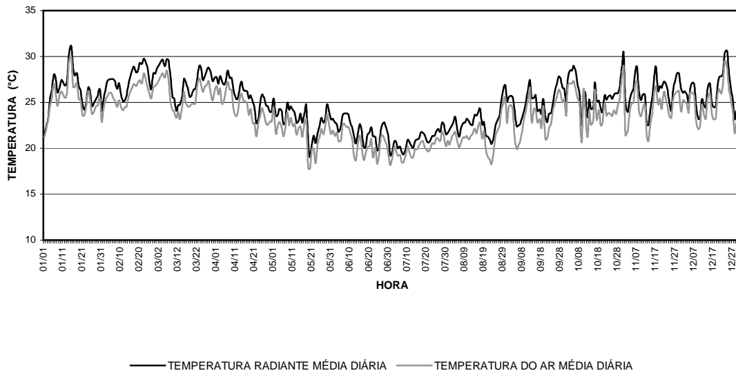
GRÁFICO 57: Gráfico das temperaturas médias diárias do ar e radiante para a sala 12 do bloco 01 para o ano meteorológico típico, gerado a partir da base de dados TMY ( Typical Meteorological Year ) para o município de Belo Horizonte.
