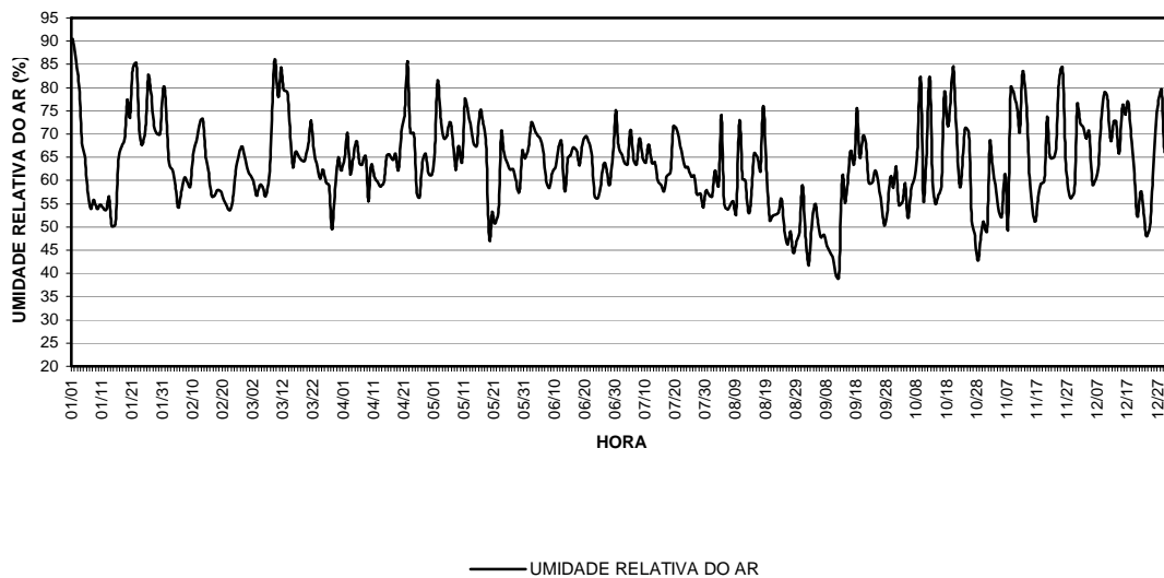
GRÁFICO 52: Gráfico das médias diárias da umidade relativa do ar para a sala 08 do bloco 01 para o ano meteorológico típico, gerado a partir da base de dados TMY ( Typical Meteorological Year ) para o município de Belo Horizonte.
