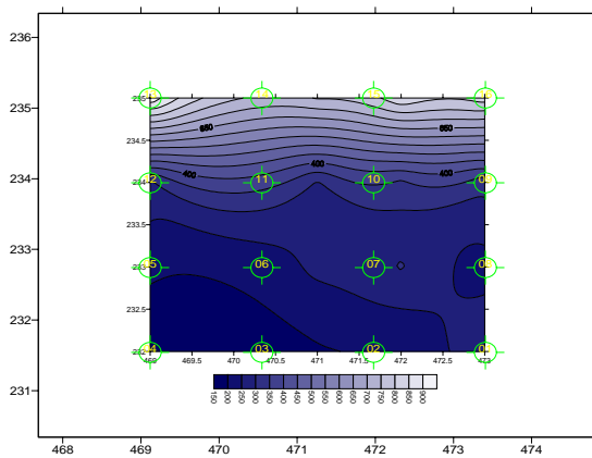
GRÁFICO 20: Iluminância da sala 03 para o dia 11/07/06 às 10:24 horas gerado c/ dados de medição – céu claro. FONTE: Elaborado pela autora.
