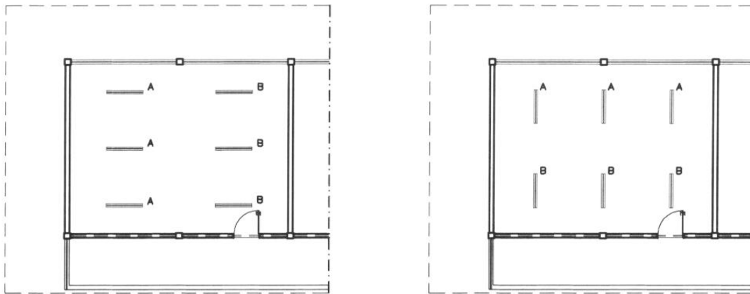
FIGURA 08: Projeto Luminotécnico atual e proposta de retrofit .
