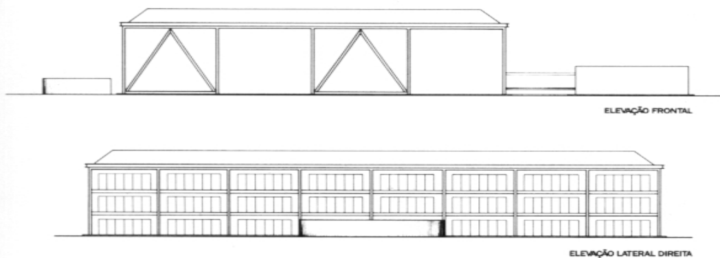
FIGURA 44: Elevação Frontal e Elevação lateral direita.
