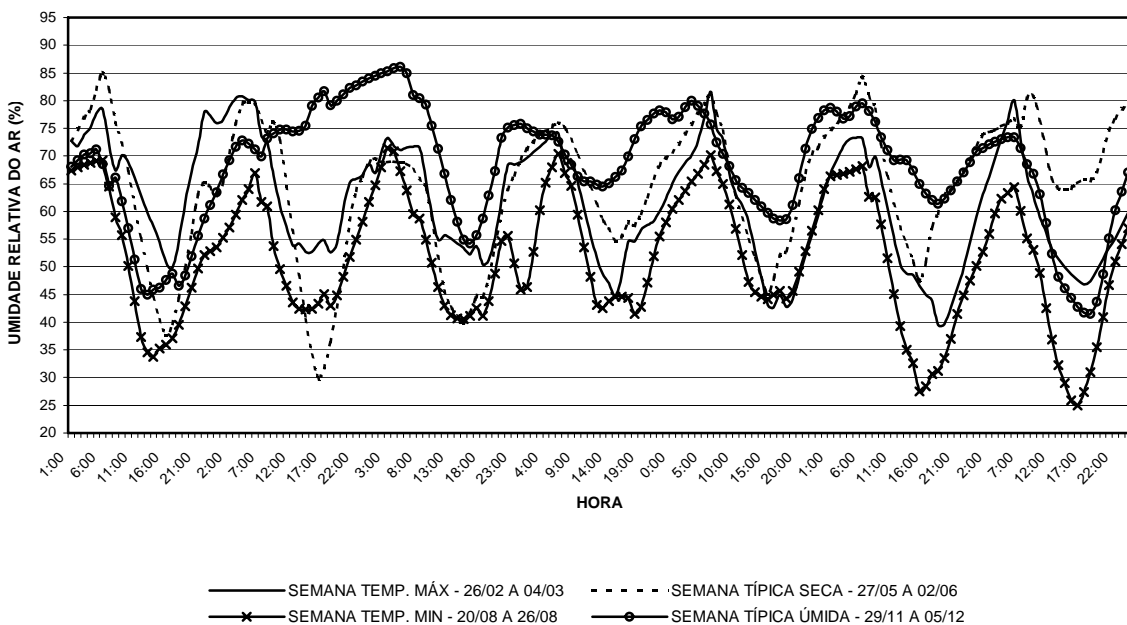
GRÁFICO 48: Gráfico de umidade relativa do ar para a sala 08 do bloco 01 para as semanas de temperaturas máximas e mínimas, e para as semanas típicas do período seco e do período úmido, gerado a partir da base de dados TMY ( Typical Meteorological Year ) para o município de Belo Horizonte. FONTE: Elaborado pela autora a partir do software Excel® com dados gerados pelo Energyplus ®.
