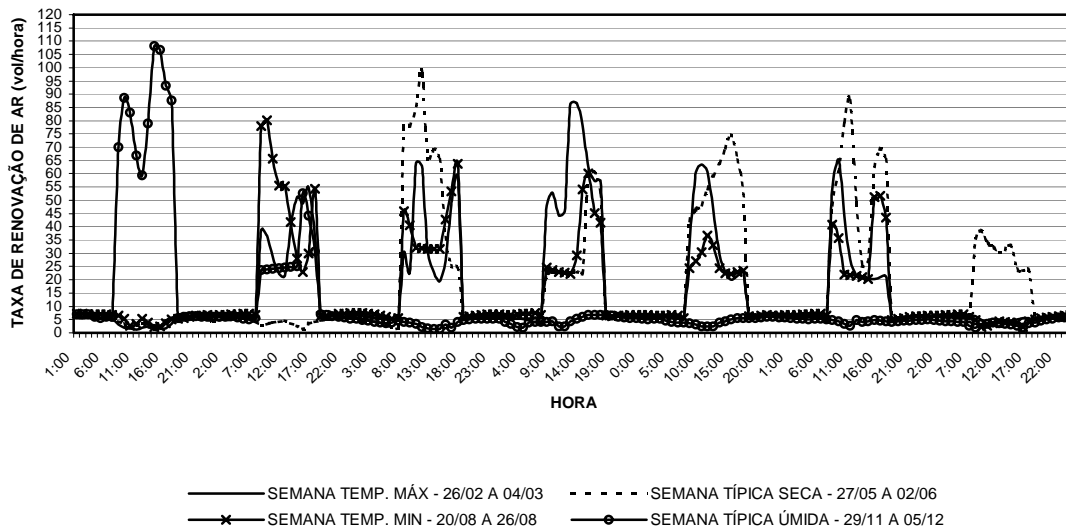
GRÁFICO 56: Gráfico da taxa de renovação de ar para a sala 12 do bloco 01 para as semanas de temperaturas máximas e mínimas, e para as semanas típicas do período seco e do período úmido, gerado a partir da base de dados TMY ( Typical Meteorological Year ) para o município de Belo Horizonte. FONTE: Elaborado pela autora a partir do software Excel® com dados gerados pelo Energyplus ®.
