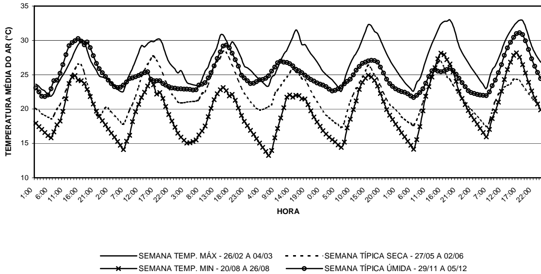
GRÁFICO 53: Gráfico de temperatura média do ar para a sala 12 do bloco 01 para as semanas de temperaturas máximas e mínimas, e para as semanas típicas do período seco e do período úmido, gerado a partir da base de dados TMY ( Typical Meteorological Year ) para o município de Belo Horizonte. FONTE: Elaborado pela autora a partir do software Excel® com dados gerados pelo Energyplus ®.
