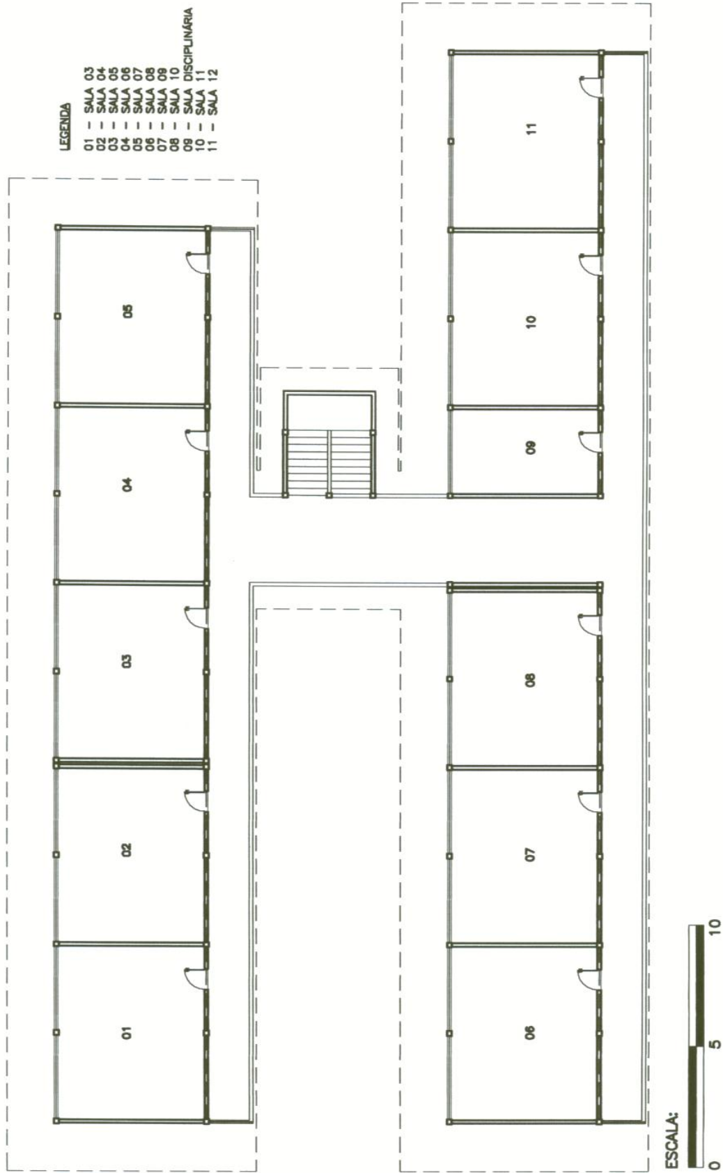
FIGURA 28: Planta geral do segundo pavimento dos blocos 01 e 02 da Escola E. Pero Vaz. FONTE: Elaborado pela autora a partir de levantamento realizado em agosto de 2005.
