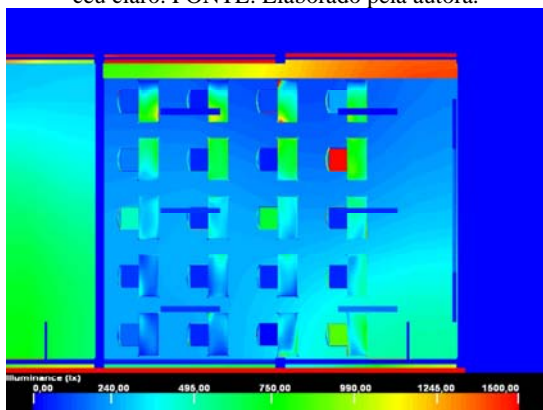
GRÁFICO 26: Iluminância da sala 12 para o dia 11/07/06 às 10:45 horas gerado a partir do modelo – céu claro. FONTE: Elaborado pela autora.
