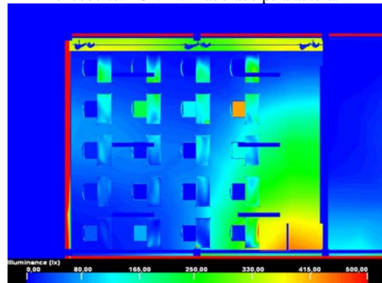
GRÁFICO 23: Iluminância da sala 03 para o dia 06/07/06 às 15:30 horas gerado a partir do modelo – céu encoberto. FONTE: Elaborado pela autora.
