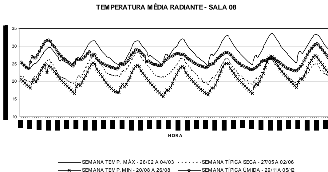
GRÁFICO 12: Temperatura média radiante para a sala 08, do bloco 01, para as semanas de temperaturas máximas e mínimas, e para as semanas típicas do período seco e do período úmido, gerado a partir da base de dados TMY ( Typical Meteorological Year ) para o município de Belo Horizonte.
