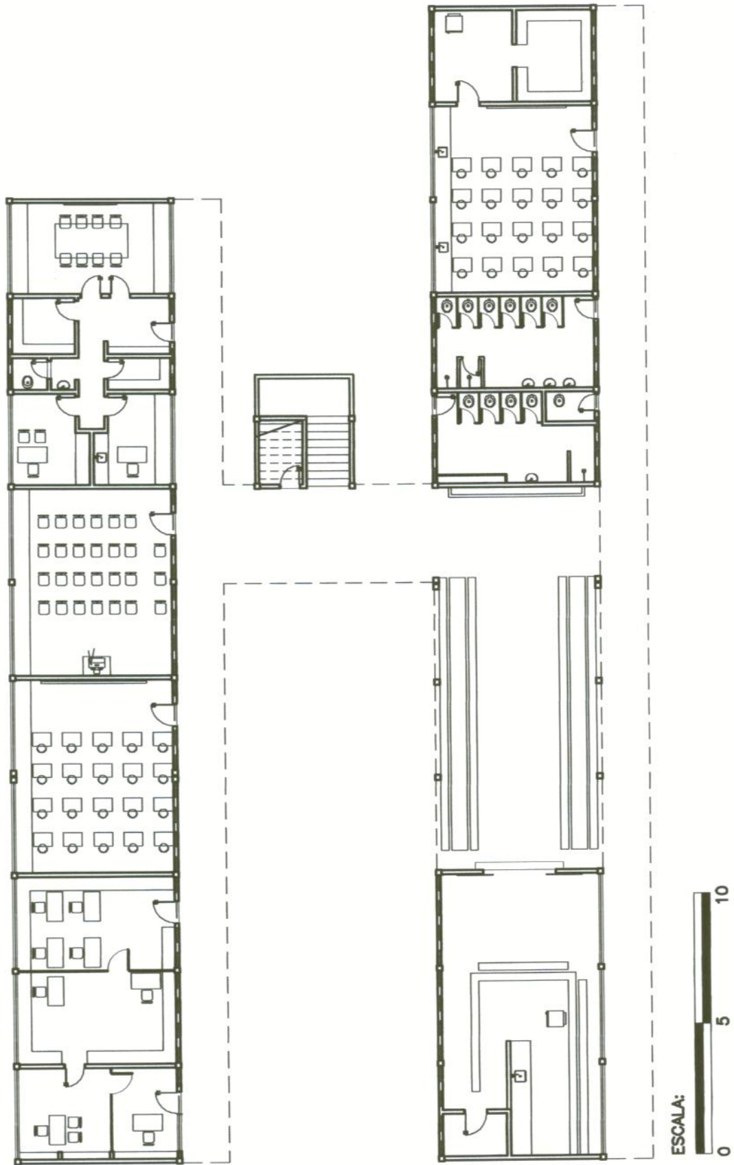
FIGURA 26: Planta de layout do primeiro pavimento dos blocos 01 e 02 da Escola E. Pero Vaz. FONTE: Elaborado pela autora a partir de levantamento realizado em agosto de 2005.
