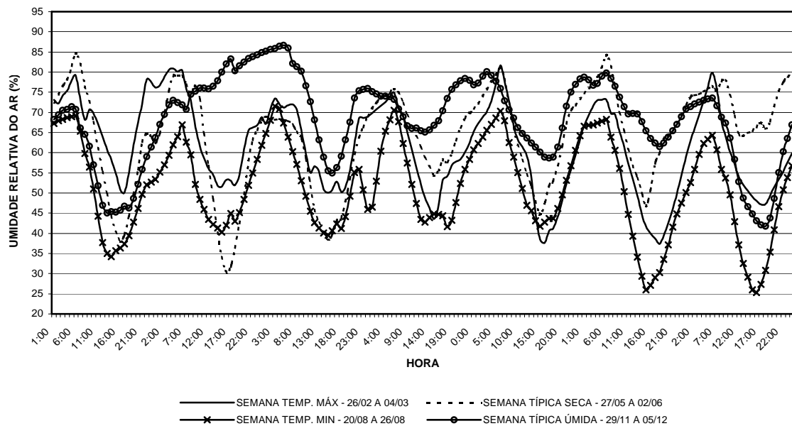
GRÁFICO 42: Gráfico de umidade relativa do ar para a sala 07 do bloco 02 para as semanas de temperaturas máximas e mínimas, e para as semanas típicas do período seco e do período úmido, gerado a partir da base de dados TMY ( Typical Meteorological Year ) para o município de Belo Horizonte. FONTE: Elaborado pela autora a partir do software Excel® com dados gerados pelo Energyplus ®.
