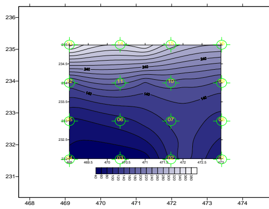
GRÁFICO 25: Iluminância da sala 12 para o dia 06/07/06 às 15:45 horas gerado c/ dados de medição – céu encoberto. FONTE: Elaborado pela autora.
