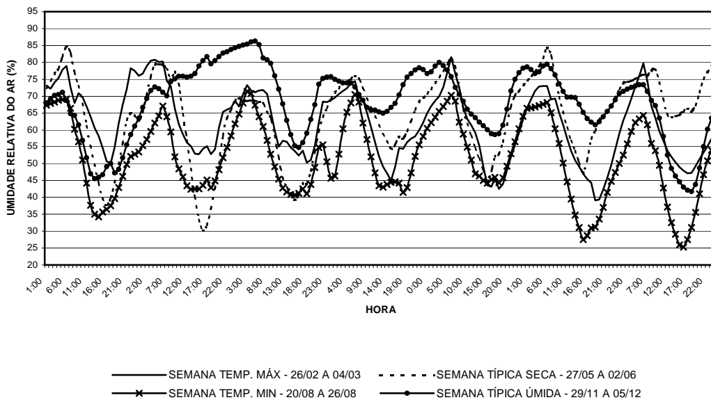
GRÁFICO 36: Gráfico de umidade relativa do ar para a sala 03 do bloco 02 para as semanas de temperaturas máximas e mínimas, e para as semanas típicas do período seco e do período úmido, gerado a partir da base de dados TMY ( Typical Meteorological Year ) para o município de Belo Horizonte.
