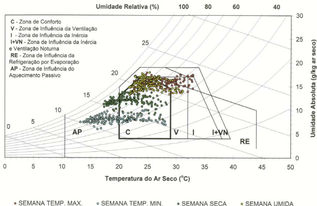
FIGURA 09: Diagrama de Givoni para o Município de Belo Horizonte.
