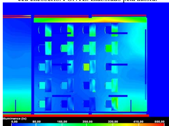
GRÁFICO 27: Iluminância da sala 12 para o dia 06/07/06 às 15:45 horas gerado a partir do modelo – céu encoberto. FONTE: Elaborado pela autora.
