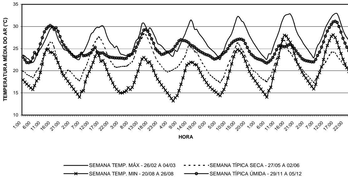
GRÁFICO 47: Gráfico de temperatura média do ar para a sala 08 do bloco 01 para as semanas de temperaturas máximas e mínimas, e para as semanas típicas do período seco e do período úmido, gerado a partir da base de dados TMY ( Typical Meteorological Year ) para o município de Belo Horizonte. FONTE: Elaborado pela autora a partir do software Excel® com dados gerados pelo Energyplus ®.
