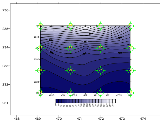
GRÁFICO 24: Iluminância da sala 12 para o dia 11/07/06 às 10:45 horas gerado c/ dados de medição – céu claro. FONTE: Elaborado pela autora.
