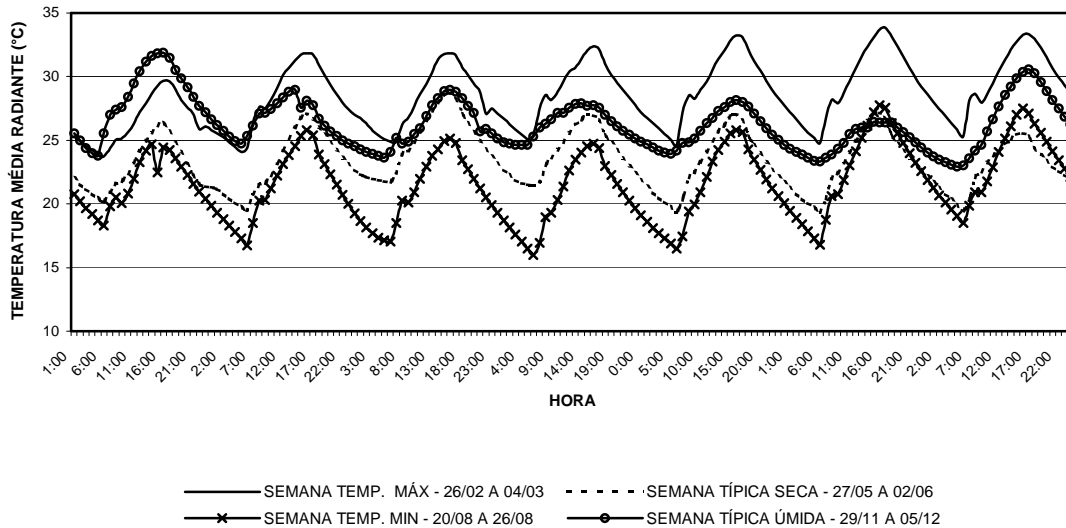
GRÁFICO 55: Gráfico de temperatura média radiante para a sala 12 do bloco 01 para as semanas de temperaturas máximas e mínimas, e para as semanas típicas do período seco e do período úmido, gerado a partir da base de dados TMY ( Typical Meteorological Year ) para o município de Belo Horizonte. FONTE: Elaborado pela autora a partir do software Excel® com dados gerados pelo Energyplus ®.
