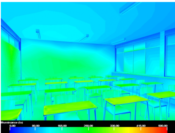
GRÁFICO 64: Iluminância em perspectiva da sala 12 no período da noite gerado a partir do modelo. FONTE: Elaborado pela autora.
