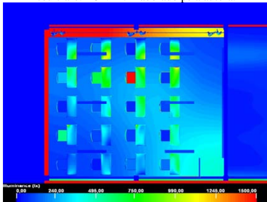
GRÁFICO 22: Iluminância da sala 03 para o dia 11/07/06 às 10:24 horas gerado a partir do modelo – céu claro. FONTE: Elaborado pela autora.
