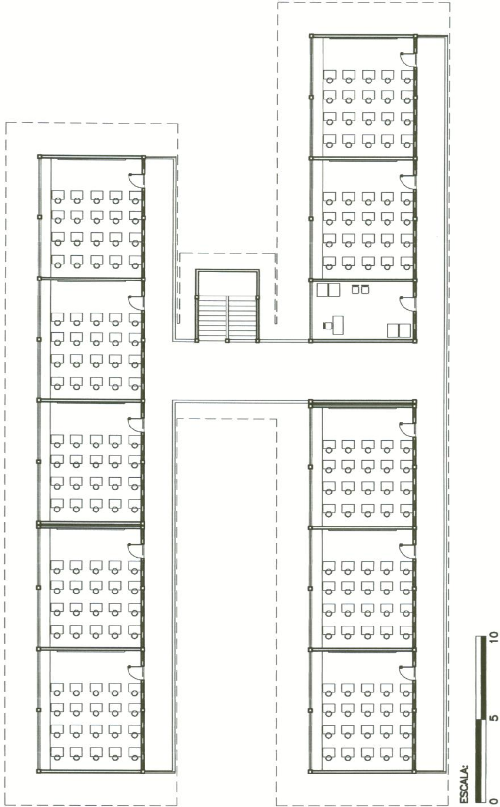
FIGURA 29: Planta de layout do segundo pavimento dos blocos 01 e 02 da Escola E. Pero Vaz. FONTE: Elaborado pela autora a partir de levantamento realizado em agosto de 2005.
