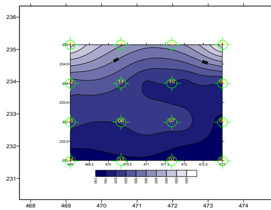
GRÁFICO 21: Iluminância da sala 03 para o dia 06/07/06 às 15:30 gerado c/ dados de medição – céu encoberto. FONTE: Elaborado pela autora.
