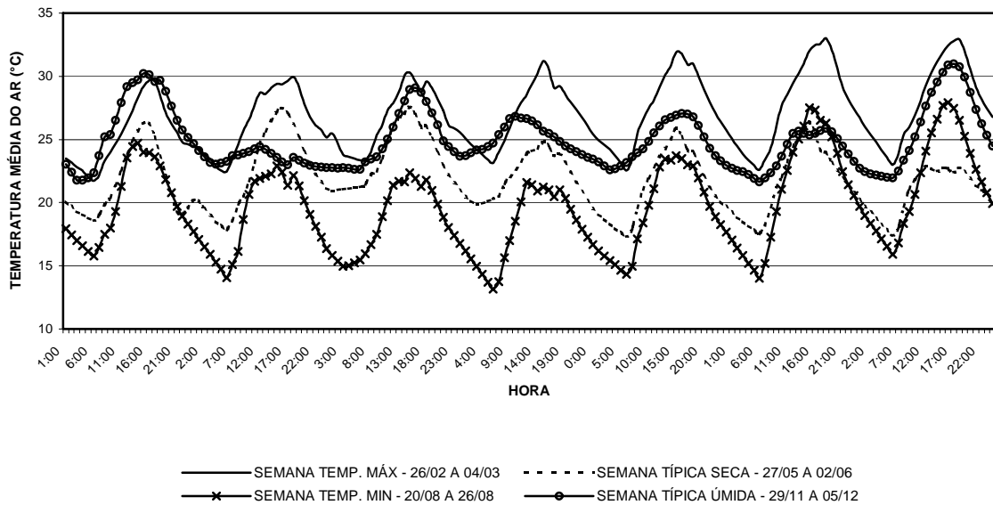
GRÁFICO 41: Gráfico de temperatura média do ar para a sala 07 do bloco 02 para as semanas de temperaturas máximas e mínimas, e para as semanas típicas do período seco e do período úmido, gerado a partir da base de dados TMY ( Typical Meteorological Year ) para o município de Belo Horizonte. FONTE: Elaborado pela autora a partir do software Excel® com dados gerados pelo Energyplus ®.
