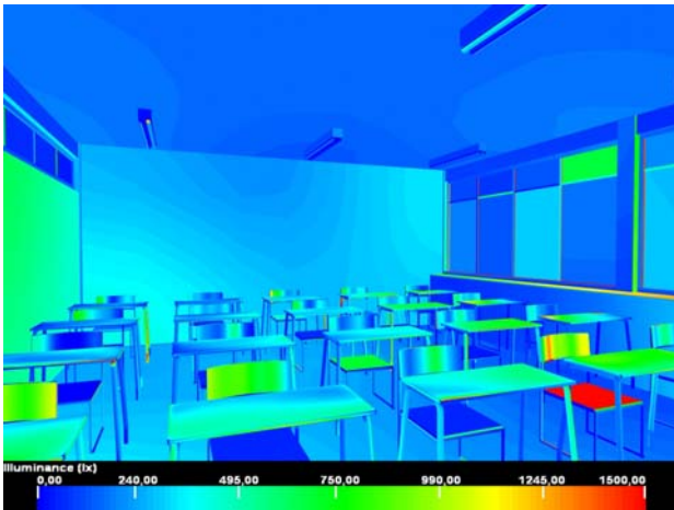
GRÁFICO 62: Iluminância em perspectiva da sala 12 pela manhã gerado a partir do modelo – céu claro. FONTE: Elaborado pela autora.
