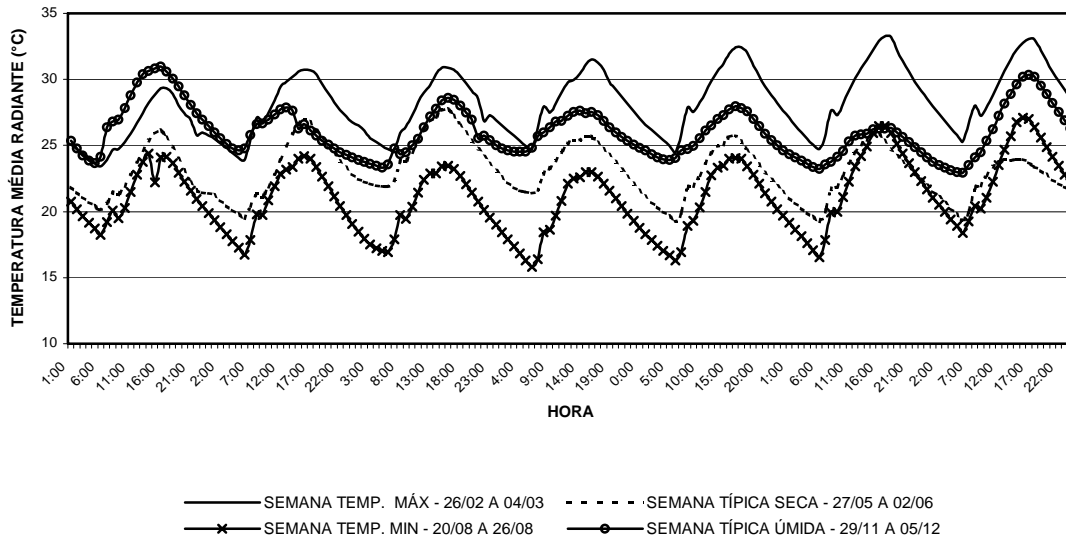
GRÁFICO 43: Gráfico de temperatura média radiante para a sala 07 do bloco 02 para as semanas de temperaturas máximas e mínimas, e para as semanas típicas do período seco e do período úmido, gerado a partir da base de dados TMY ( Typical Meteorological Year ) para o município de Belo Horizonte. FONTE: Elaborado pela autora a partir do software Excel® com dados gerados pelo Energyplus ®.
