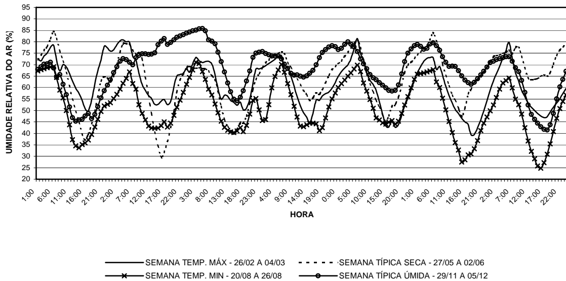
GRÁFICO 54: Gráfico de umidade relativa do ar para a sala 12 do bloco 01 para as semanas de temperaturas máximas e mínimas, e para as semanas típicas do período seco e do período úmido, gerado a partir da base de dados TMY ( Typical Meteorological Year ) para o município de Belo Horizonte. FONTE: Elaborado pela autora a partir do software Excel® com dados gerados pelo Energyplus ®.
