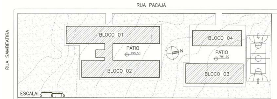
FIGURA 23: Planta de Implantação da Escola E. Pero Vaz. FONTE: Elaborado pela autora a partir de levantamento realizado em agosto de 2005.
