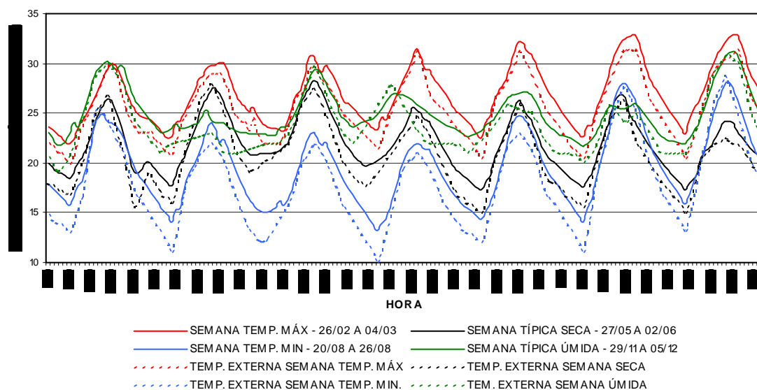
GRÁFICO 14: Temperatura média do ar e temperaturas externas para a sala 08, do bloco 01, para as semanas de temperaturas máximas e mínimas, para as semanas típicas do período seco e do período úmido, gerado a partir da base de dados TMY para o município de Belo Horizonte.
