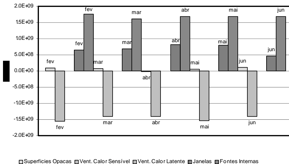
GRÁFICO 15-A: Balanço térmico da sala 08 para os meses letivos do 1º semestre do ano simulado. FONTE: Elaborado pela autora a partir do software Excel® com dados gerados pelo Energyplus ®.
