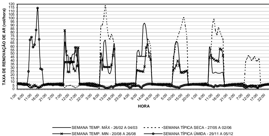
GRÁFICO 38: Gráfico da taxa de renovação de ar para a sala 03 do bloco 02 para as semanas de temperaturas máximas e mínimas, e para as semanas típicas do período seco e do período úmido, gerado a partir da base de dados TMY ( Typical Meteorological Year ) para o município de Belo Horizonte. FONTE: Elaborado pela autora a partir do software Excel® com dados gerados pelo Energyplus ®.
