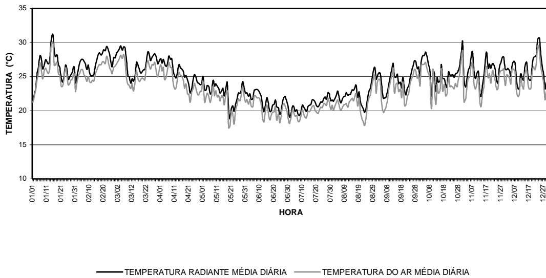
GRÁFICO 51: Gráfico das temperaturas médias diárias do ar e radiante para a sala 08 do bloco 01 para o ano meteorológico típico, gerado a partir da base de dados TMY ( Typical Meteorological Year ) para o município de Belo Horizonte.
