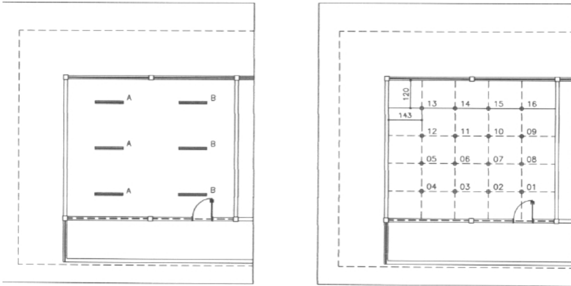
FIGURA 35: Planta Luminotécnica da sala 03 e localização dos pontos de medição.
