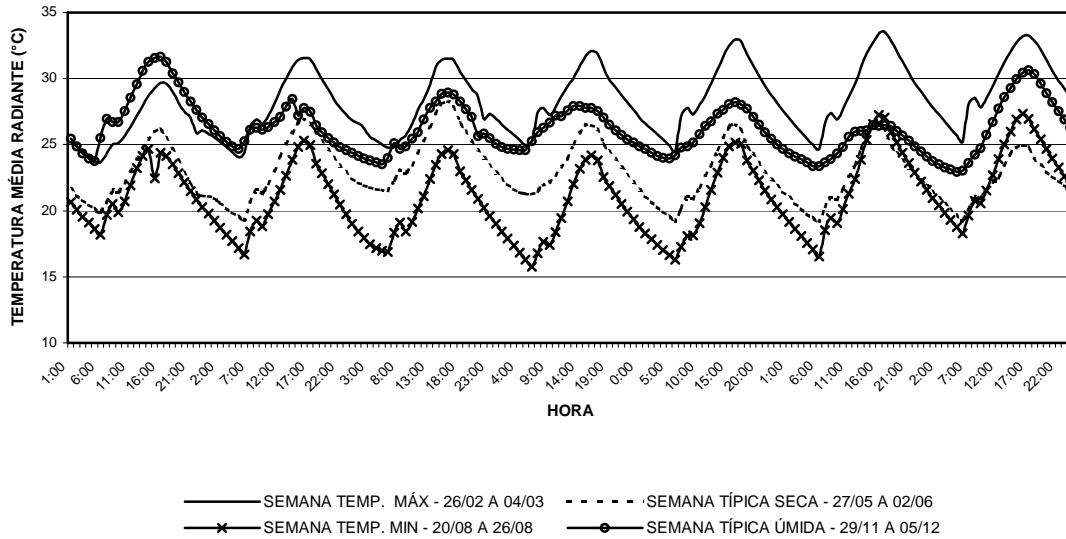
GRÁFICO 49: Gráfico de temperatura média radiante para a sala 08 do bloco 01 para as semanas de temperaturas máximas e mínimas, e para as semanas típicas do período seco e do período úmido, gerado a partir da base de dados TMY ( Typical Meteorological Year ) para o município de Belo Horizonte. FONTE: Elaborado pela autora a partir do software Excel® com dados gerados pelo Energyplus ®.
