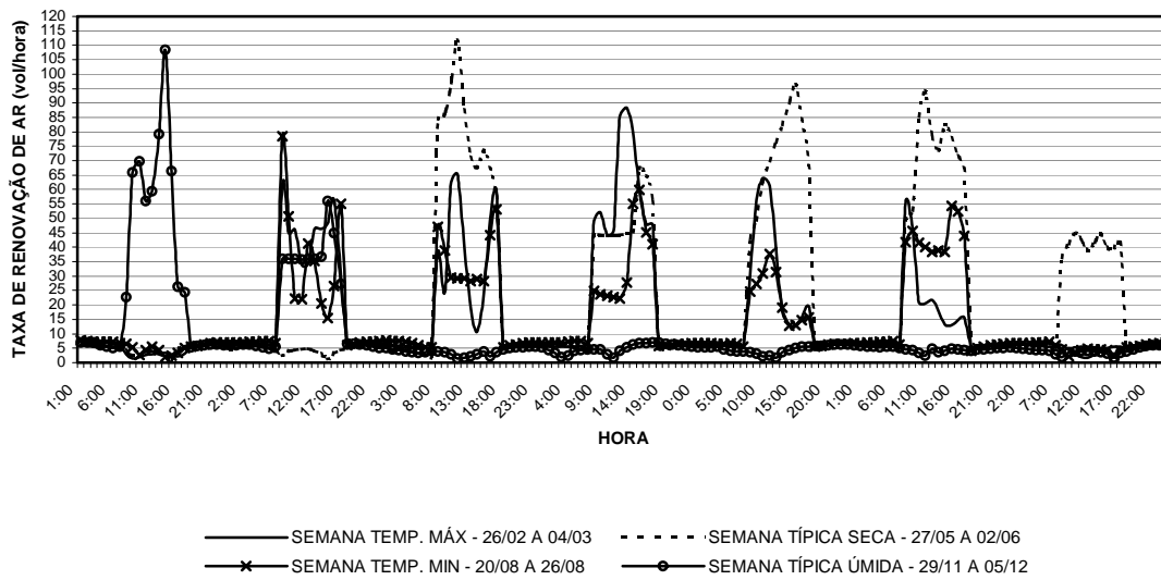
GRÁFICO 44: Gráfico da taxa de renovação de ar para a sala 07 do bloco 02 para as semanas de temperaturas máximas e mínimas, e para as semanas típicas do período seco e do período úmido, gerado a partir da base de dados TMY ( Typical Meteorological Year ) para o município de Belo Horizonte. FONTE: Elaborado pela autora a partir do software Excel® com dados gerados pelo Energyplus ®.
