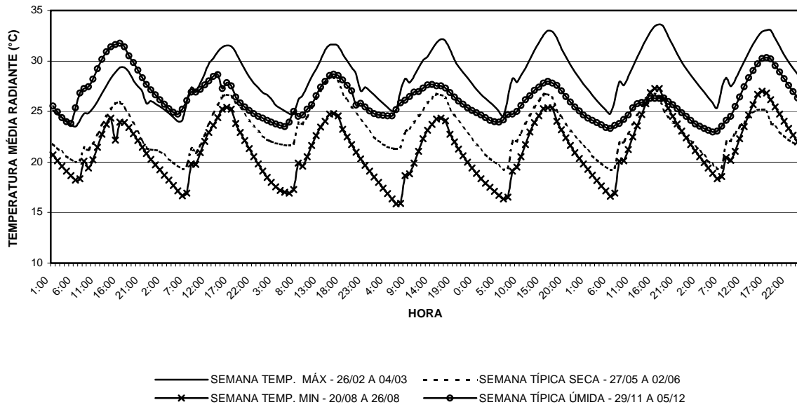
GRÁFICO 37: Gráfico de temperatura média radiante para a sala 03 do bloco 02 para as semanas de temperaturas máximas e mínimas, e para as semanas típicas do período seco e do período úmido, gerado a partir da base de dados TMY ( Typical Meteorological Year ) para o município de Belo Horizonte. FONTE: Elaborado pela autora a partir do software Excel® com dados gerados pelo Energyplus ®.
