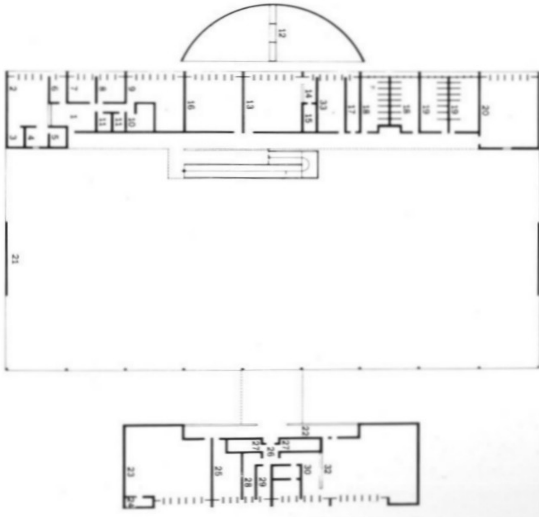
FIGURA 43: Planta do Pavimento Térreo do Padrão NEEC III: 1- administração; 2- secretaria, 3- arquivo, 4- mecanografia, 5- almoxarifado, 6- tesouraria, 7- diretoria, 8- supervisora, 9- sl professores, 10- atendimento, 11- I.S., 12- jardim, 13- laboratório, 14- sl preparo, 15- estoque, 16- sl recursos especializados, 17- dep. esportes, 18- vestiários, 19- I.S., 20- sl recursos gerais, 21- varandão, 22- circulação, 23- biblioteca, 24- depósito, 25- enfermaria, 26- circulação, 27- I.S., 28- zeladoria, 29- área de serviço, 30- despensa, 31- refeitório, 32- depósito cadeiras.
