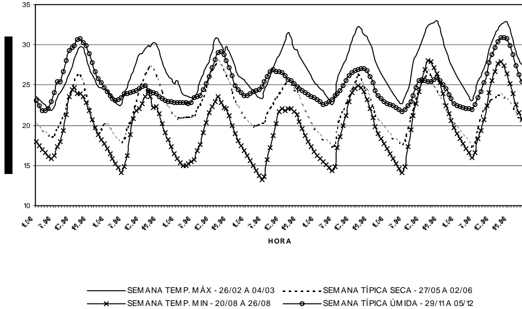
GRÁFICO 35: Gráfico de temperatura média do ar para a sala 03 do bloco 02 para as semanas de temperaturas máximas e mínimas, e para as semanas típicas do período seco e do período úmido, gerado a partir da base de dados TMY ( Typical Meteorological Year ) para o município de Belo Horizonte.
