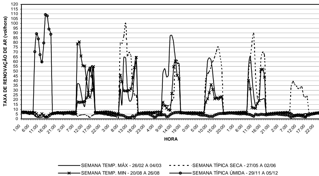
GRÁFICO 50: Gráfico da taxa de renovação de ar para a sala 08 do bloco 01 para as semanas de temperaturas máximas e mínimas, e para as semanas típicas do período seco e do período úmido, gerado a partir da base de dados TMY ( Typical Meteorological Year ) para o município de Belo Horizonte. FONTE: Elaborado pela autora a partir do software Excel® com dados gerados pelo Energyplus ®.
