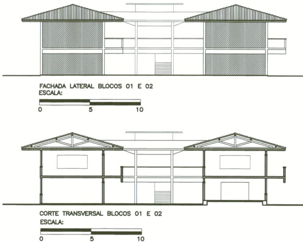
FIGURA 24: Fachada Lateral e Corte Transversal da Escola E. Pero Vaz. FONTE: Elaborado pela autora a partir de levantamento realizado em agosto de 2005.
