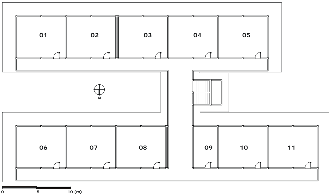
FIGURA 03: Planta 2º pavto Padrão Carpe – 01 à 08, 10 e 11 salas de aula; 09 orientação educacional.
