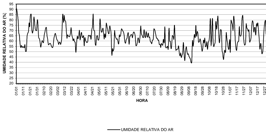
GRÁFICO 58: Gráfico das médias diárias da umidade relativa do ar para a sala 12 do bloco 01 para o ano meteorológico típico, gerado a partir da base de dados TMY ( Typical Meteorological Year ) para o município de Belo Horizonte.
