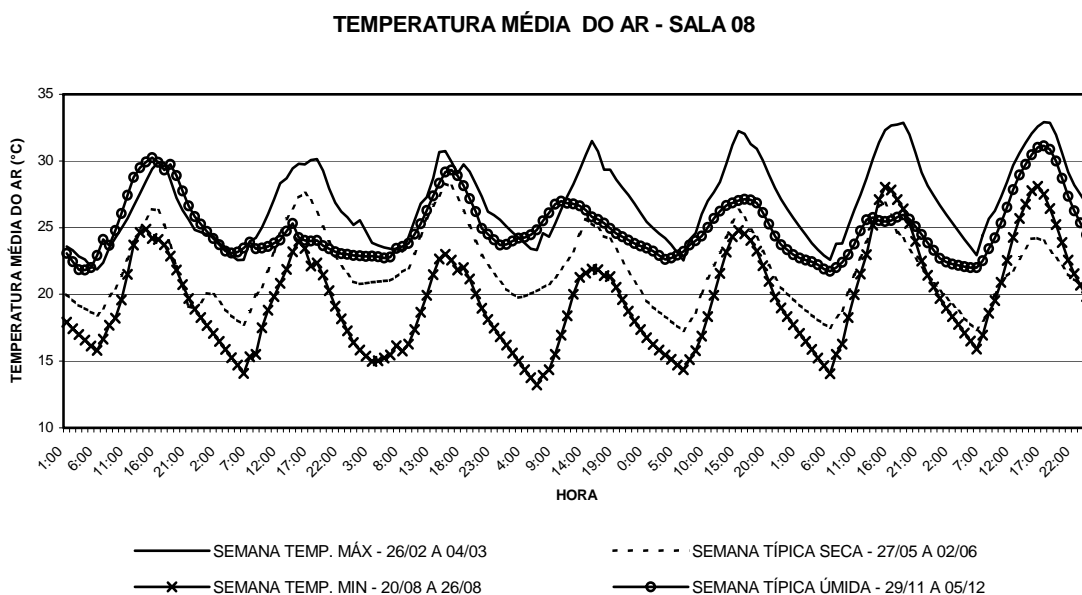
GRÁFICO 11: Temperatura média do ar para a sala 08, do bloco 01, para as semanas de temperaturas máximas e mínimas, e para as semanas típicas do período seco e do período úmido, gerado a partir da base de dados TMY ( Typical Meteorological Year ) para o município de Belo Horizonte.
