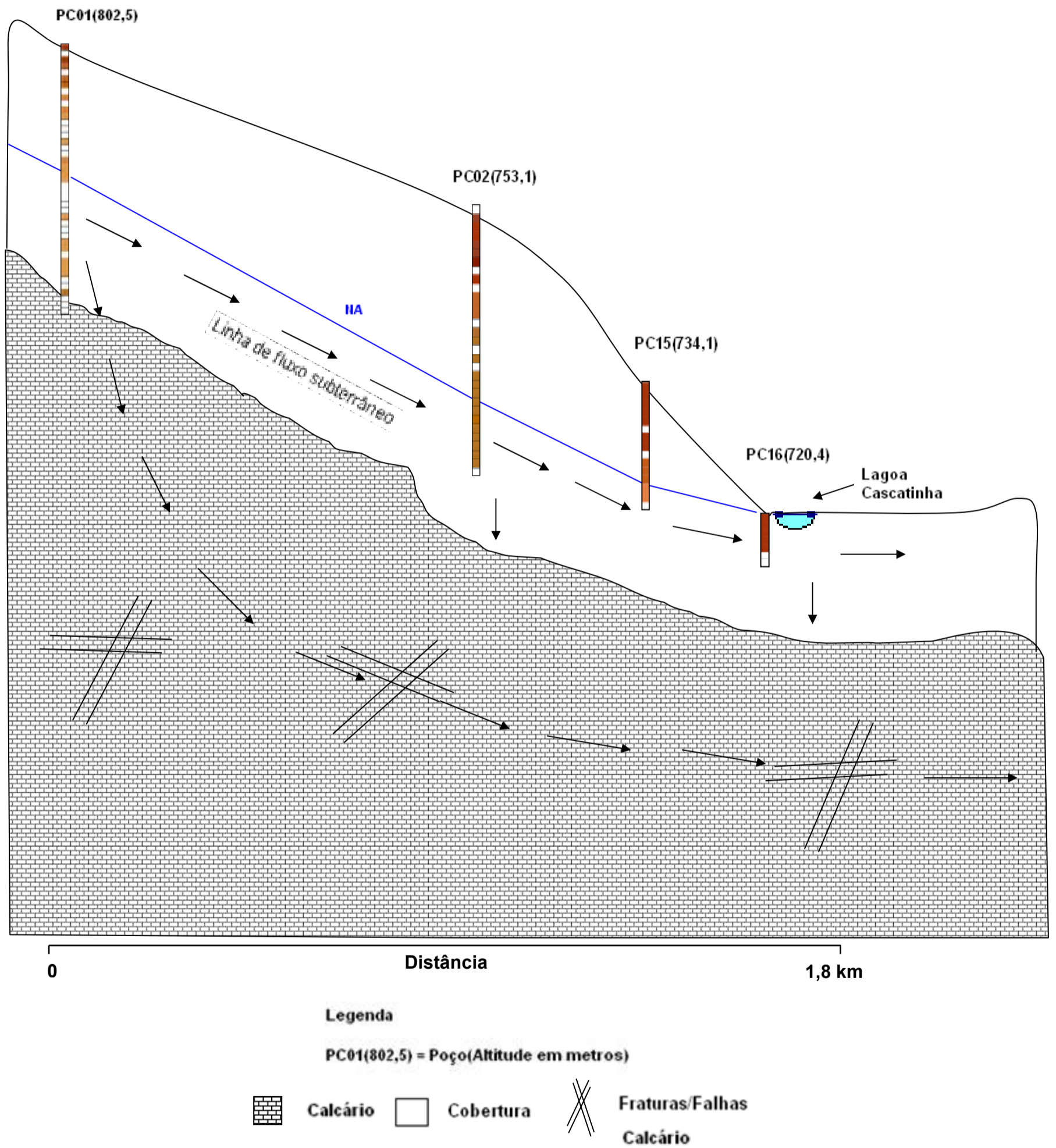
Figura 7-63 – Perfil 6: Perfil hidrogeológico esquemático entre os poços PC01 e o PC16
