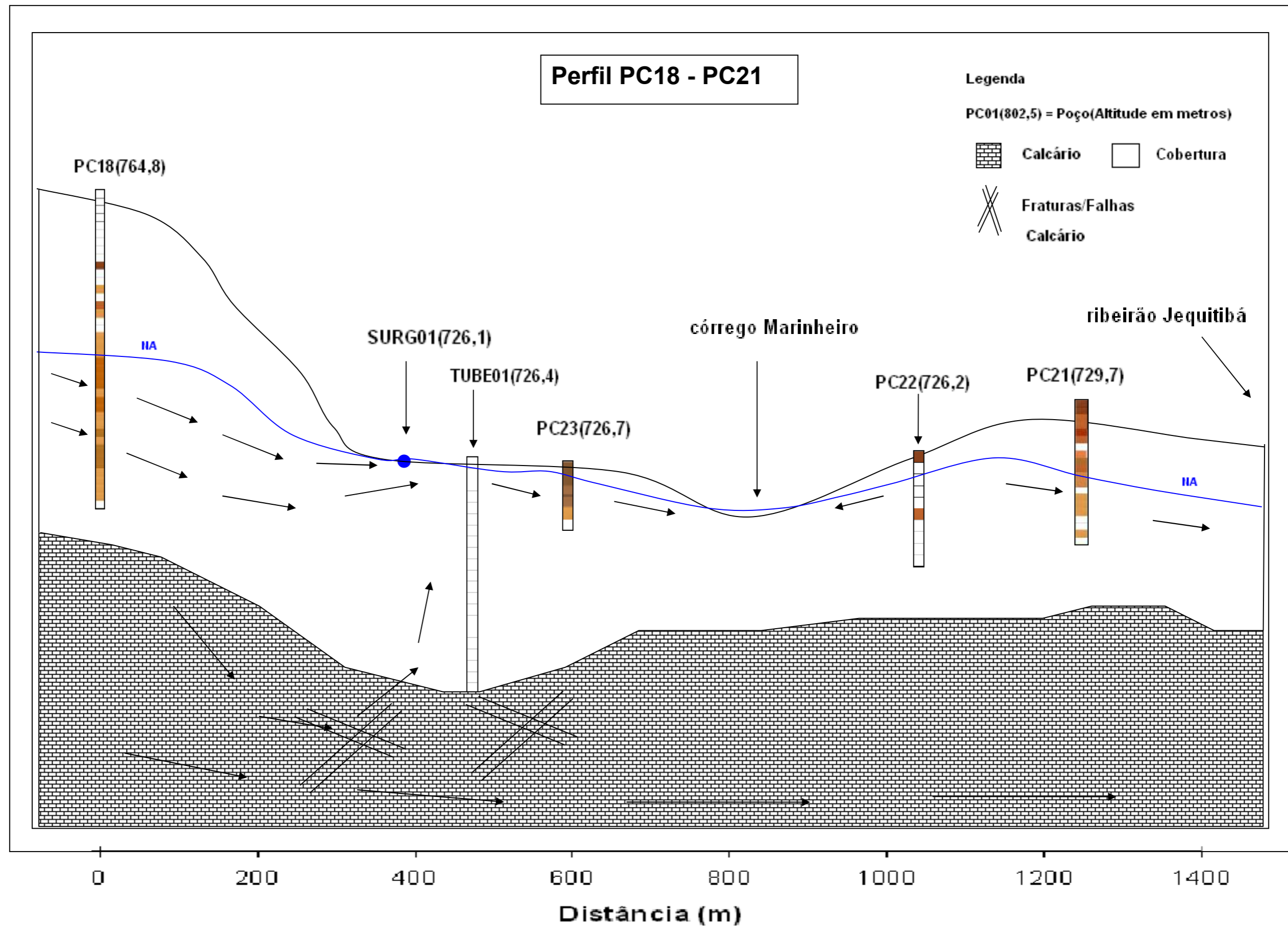
Figura 7-61 - Perfil 5: Perfil hidrogeológico esquemático entre os poços PC18 e o PC21
