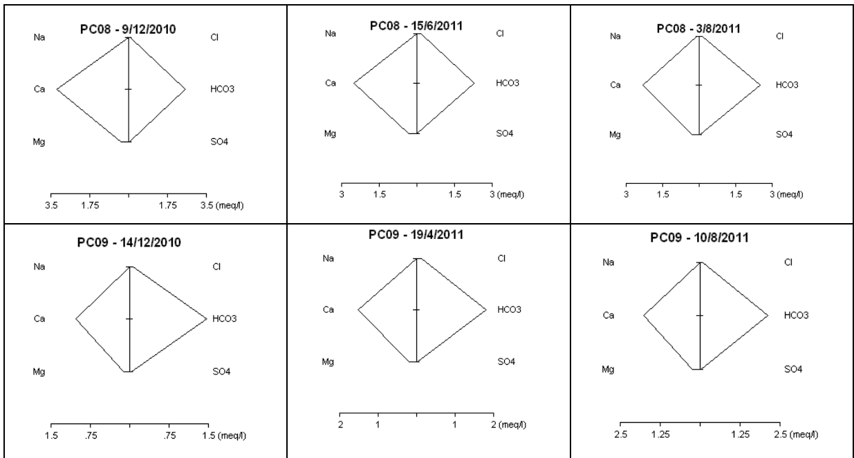
Figura 7-22 – Diagramas de Stiff para valores de medianas dos pontos dos Grupos 5 e 6
