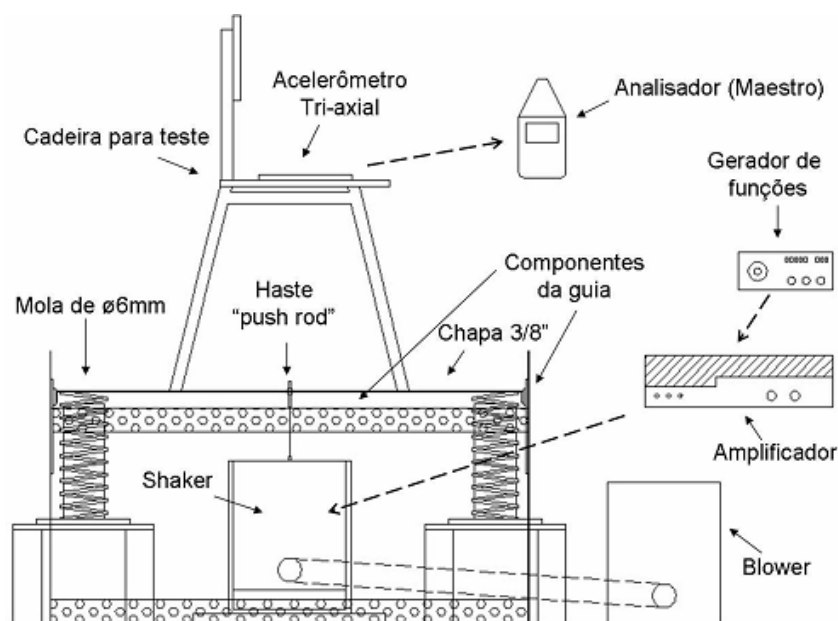
Figura 3.5 - Desenho esquemático da montagem.
