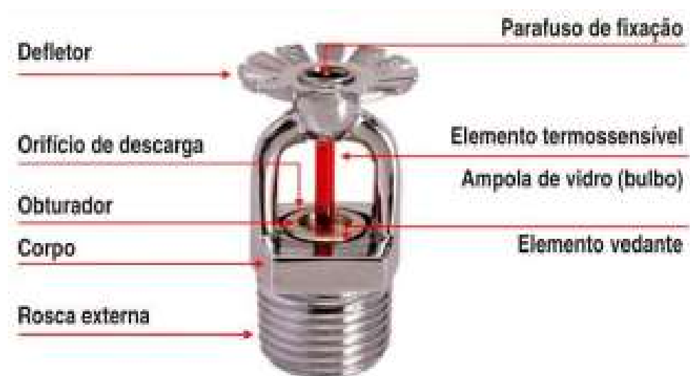
Figura 18 – Sprinkler.
